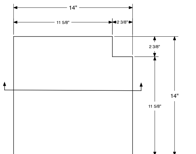
SQUARE EDGE COPING
